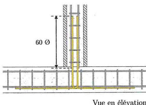
Chaînage au niveau des fondations
