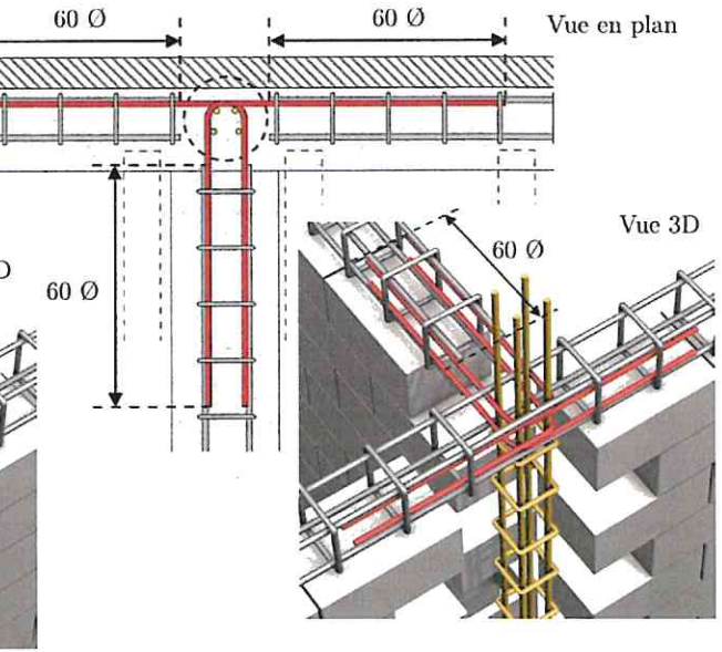
Liaison en partie courante avec équerres
