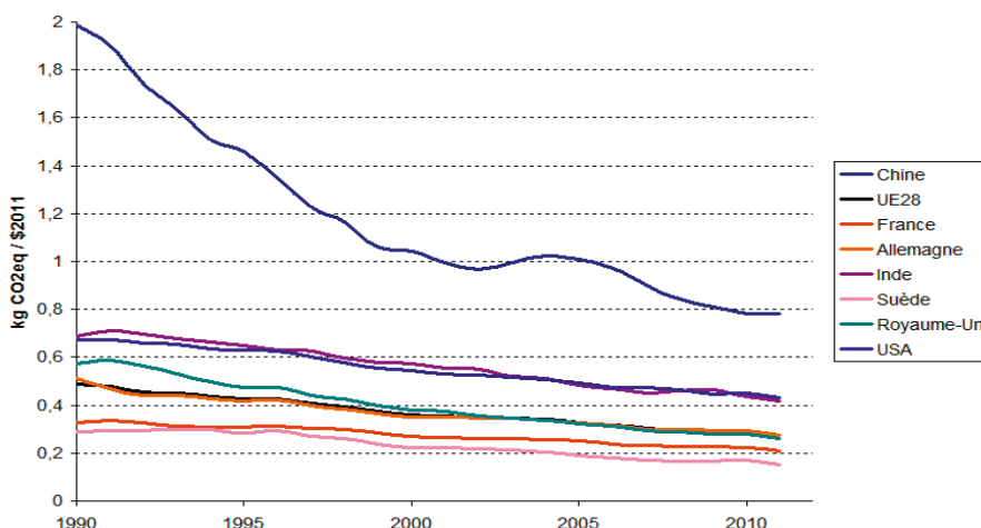
Figure 1.1 : Emissions de GES par unité de PIB (PPA). Sources : Emissions hors usage des terres (CCNUCC – sauf Chine et Inde WRI/CAIT) et PIB (Banque Mondiale)
