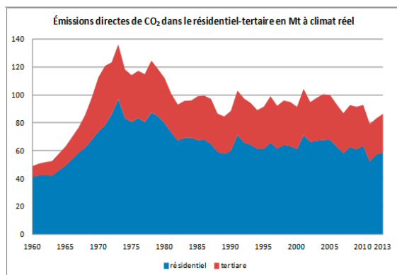
Figure 6.9 : émissions directes de CO 2 dans le résidentiel-tertiaire à climat réel
