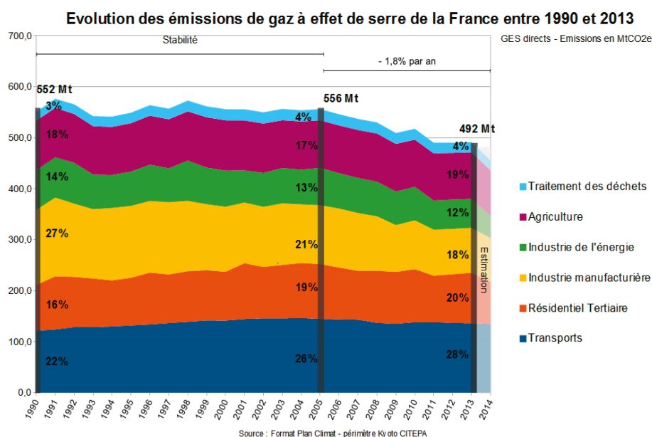
Figure 1.2 : inventaires d'émissions de gaz à effet de serre de la France (Format plan climat, périmètre Kyoto incluant la métropole et les départements et régions d'outre-mer). Source : CITEPA
