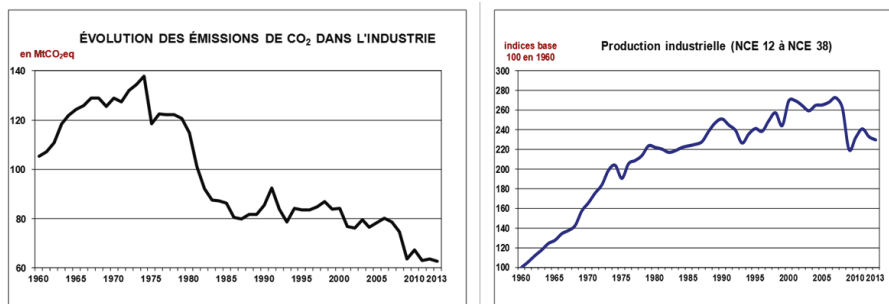
Figure 6.16 : évolution des émissions directes de GES de l'industrie liées à la consommation directe d'énergie (en Mt eq. CO 2 ) entre 1960 et 2013 (hors émissions des procédés) et évolution de la production industrielle (base 100 en 1960)
