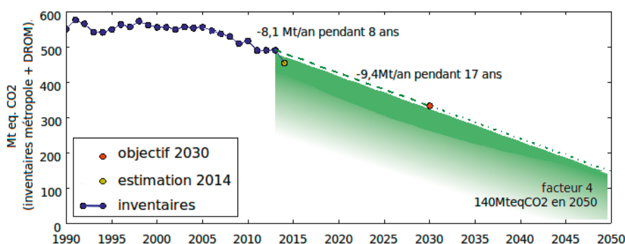
Figure 2.1 : inventaires des émissions de gaz à effet de serre (1990-2013), inventaires par approximation (2014) pour la métropole et les départements et régions d'outre-mer et objectifs d'atténuation des émissions de gaz à effet de serre de la France aux horizons 2030 et 2050. Source : CITEPA et MEDDE/DGEC
